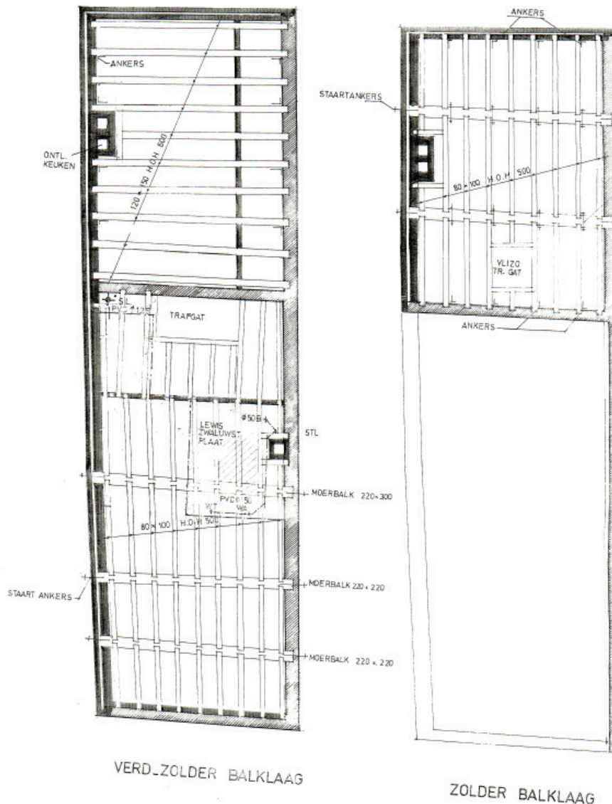
Afb. 7. De restauratietekening waarop de nieuw aan te brengen balklagen van de vloeren zijn weergegeven.
